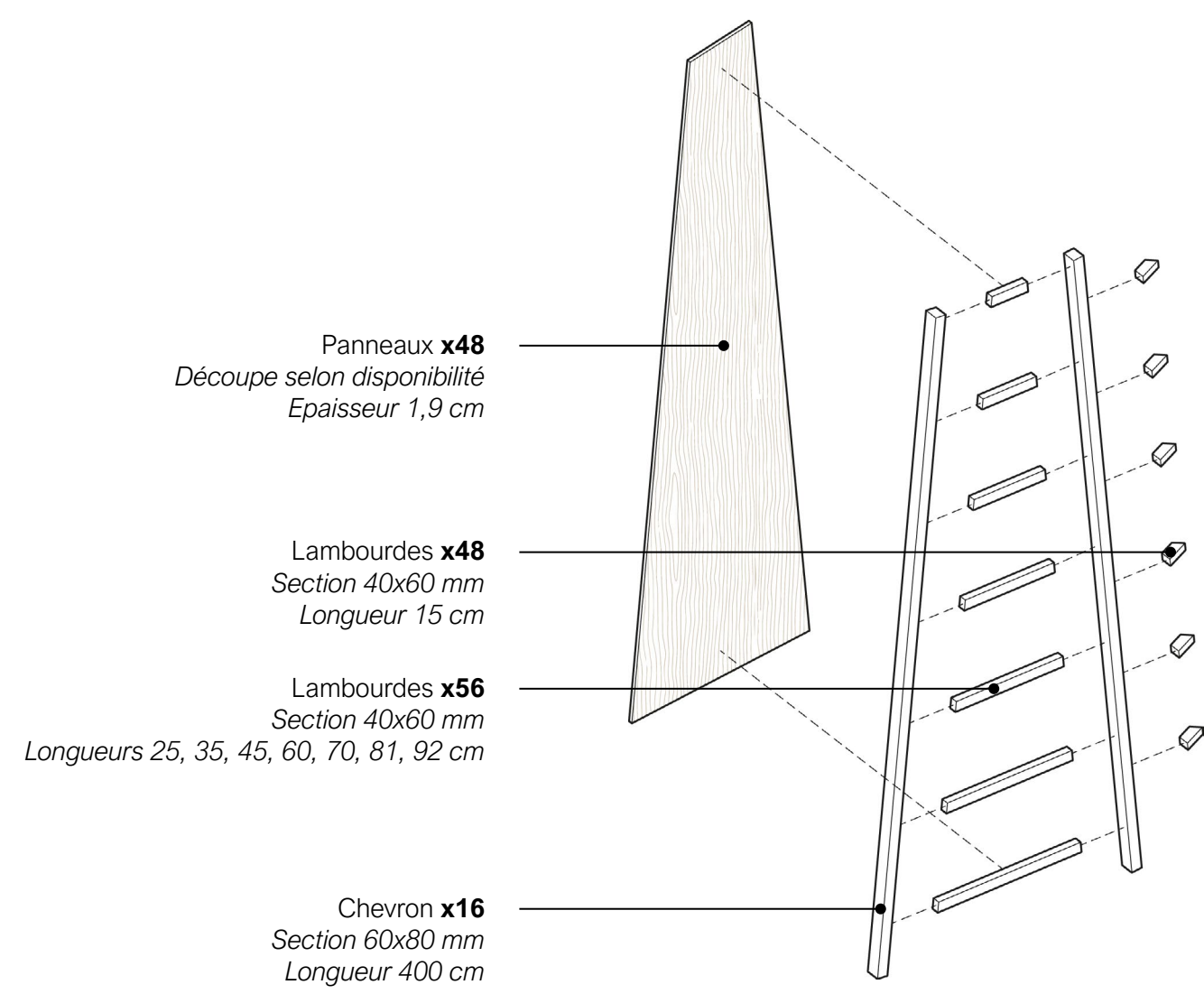
A + B Ossature + Panneaux
